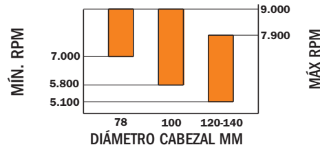
CUADRO VELOCIDADES DE CORTE INDICADAS DE LOS CABEZALES
