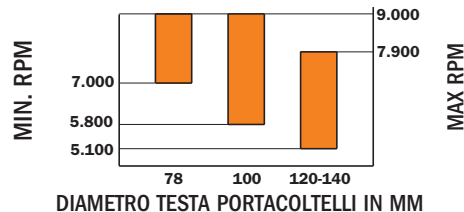
VELOCITÀ DI ROTAZIONE CONSIGLIATA DELLA TESTA
